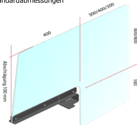
Standardabmessungen
